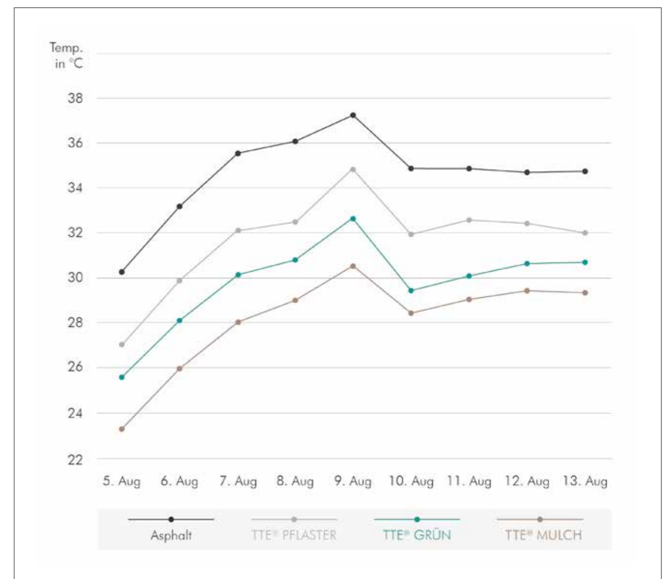
Oberflächentemperaturen verschiedener befestigter Oberflächen während einer Hitzewelle im August 2020.
