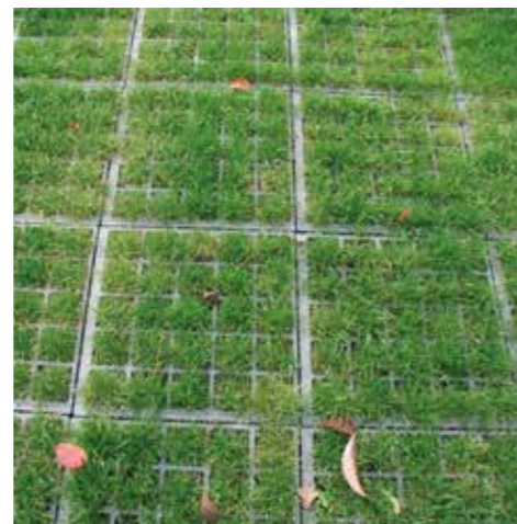
TTE® Rasengitter im Fugenversatz im Sommer 2002
